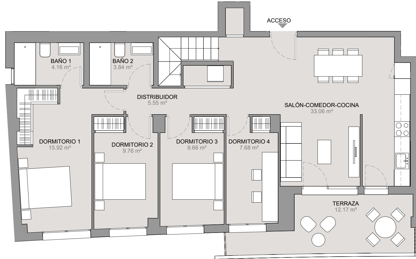
PLANTA VIVIENDA
