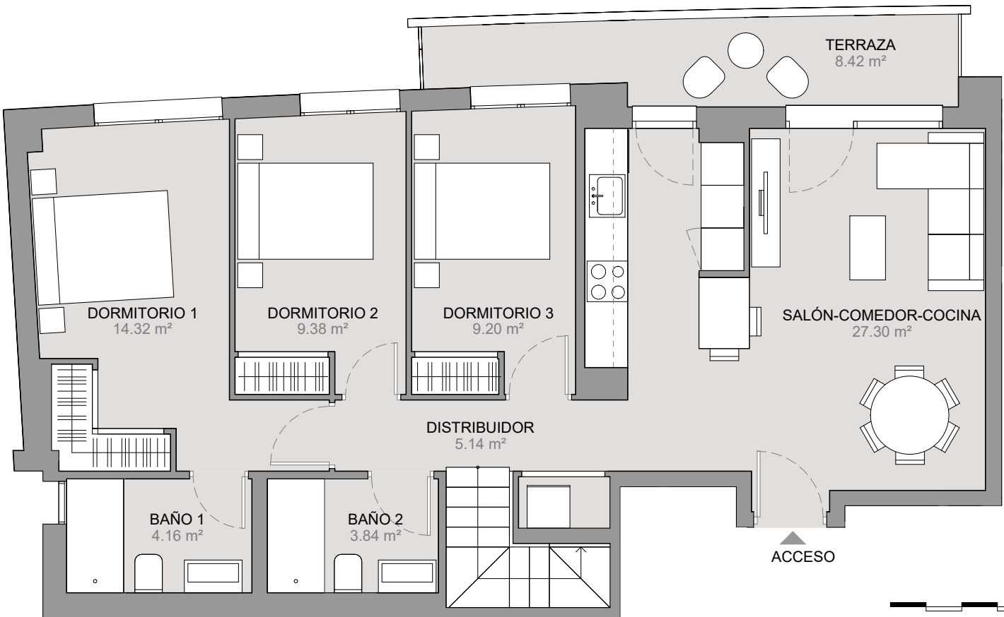
PLANTA VIVIENDA
